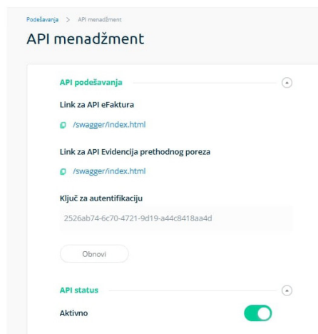
Слика бр.119 API менаџмент
